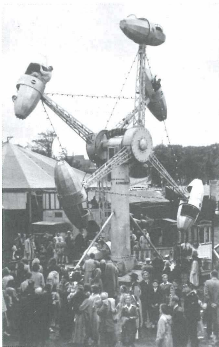
Afb. 5: Kermisattractie 'Tornado', een product van de firma Lakeman uit de jaren vijftig.
