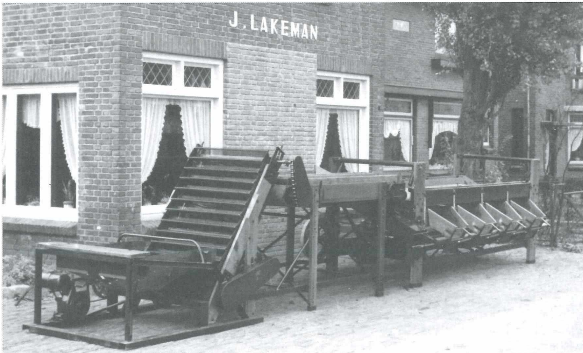
Afb. 4: Bollensortermachine van de firma Lakeman.
